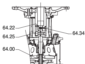
Σχ.6α Σταθεροποίηση ρότορα με απα- σφαλισμένο άξονα στην σύζευξη. (*) Σφήνα για ανύψωση του άξονα.
